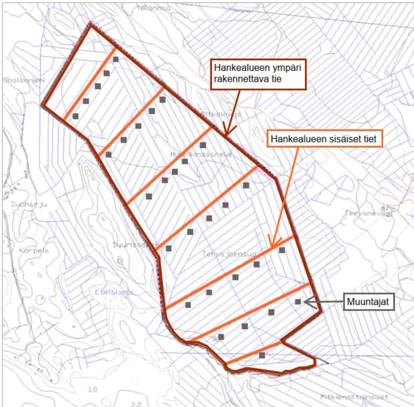
Kartta 11. Hankealueen tiestö, alustava suunnitelma. (Lähde: Envineer)
