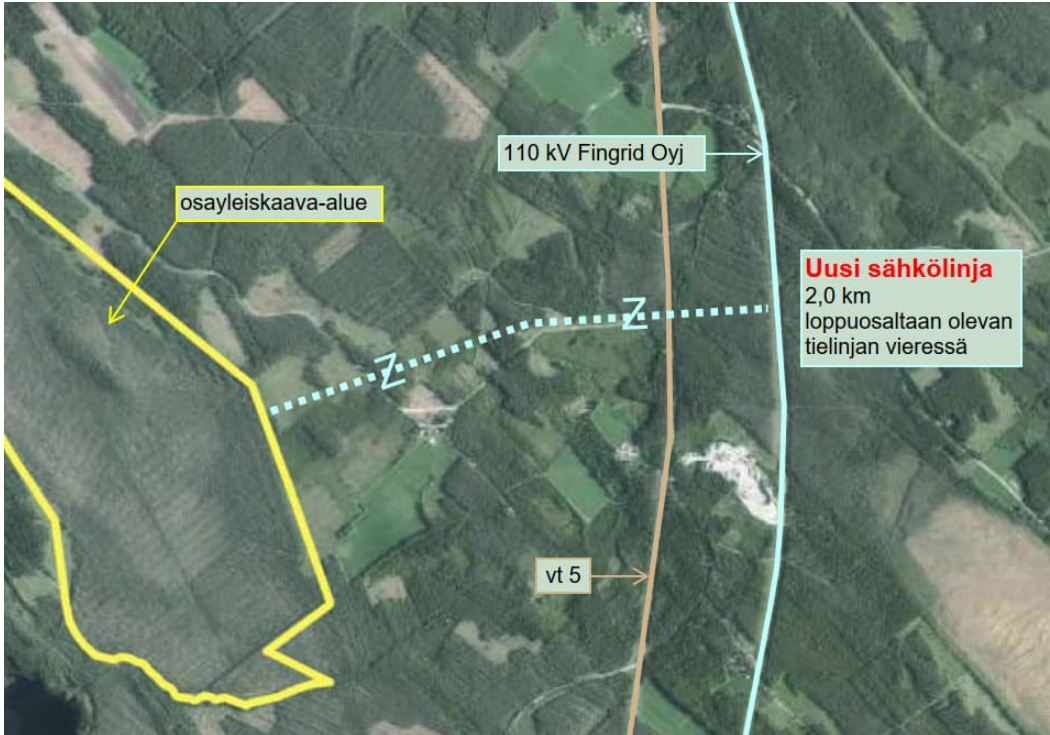
Kuva 4. Sähköliitynnän alustava linjaus. (Ilmakuva: MML)
