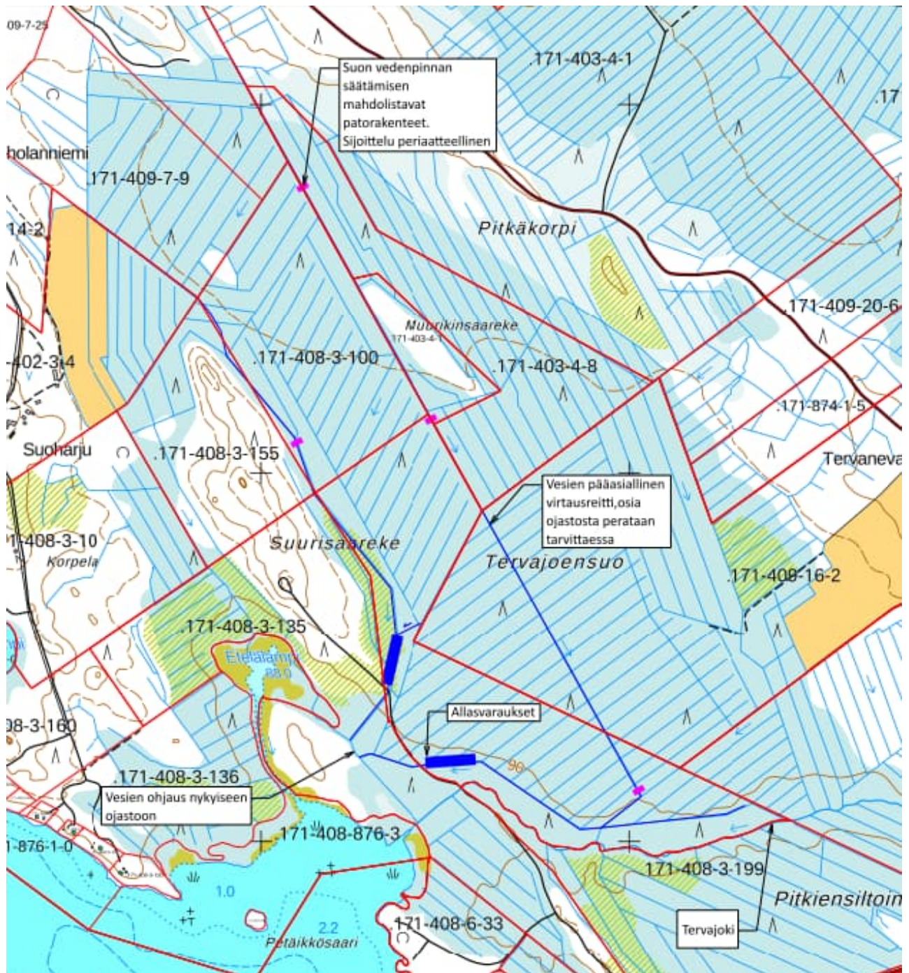
Kartta 12. Periaatepiirros aurinkovoimala-alueen vesien johtamisesta ja käsittelystä. (Periaatepiirros: Envineer, kartta: Maanmittauslaitos)
